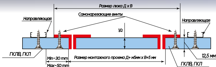
Монтажная схема люка модели «КОРNER»
